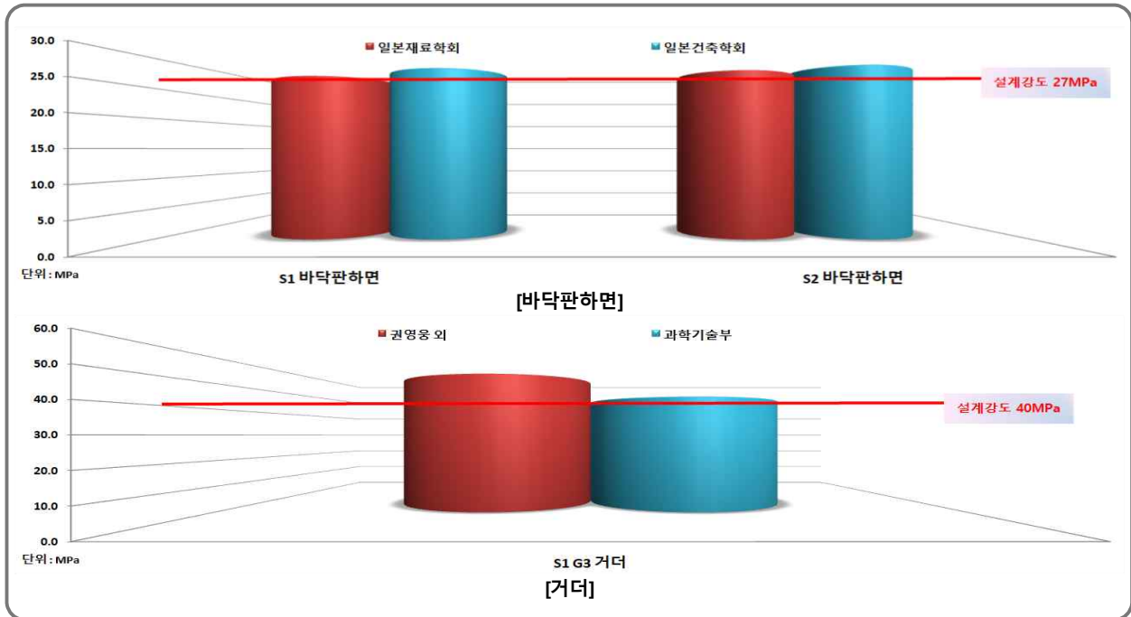
[그림 4.2.1] 반발경도법에 의한 비파괴강도 측정 결과-상부구조(바닥판하면)
