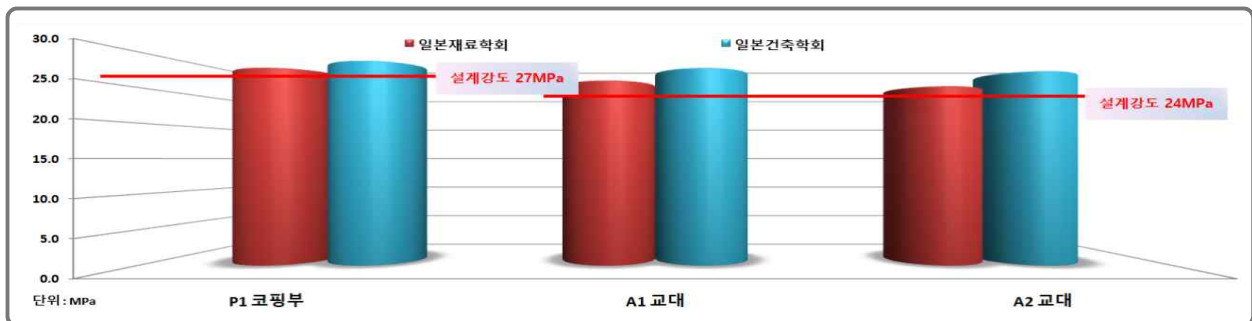
[그림 4.2.2] 반발경도법에 의한 비파괴강도 측정 결과-하부구조
